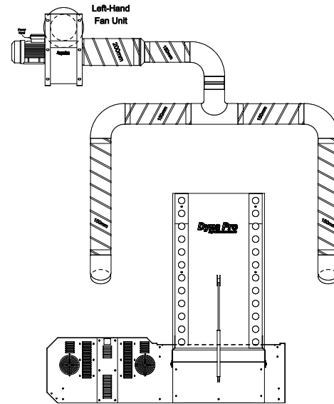
End Elevation
